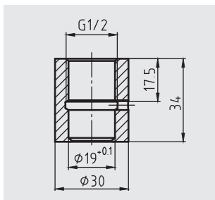
焊接套筒 G 1/2
